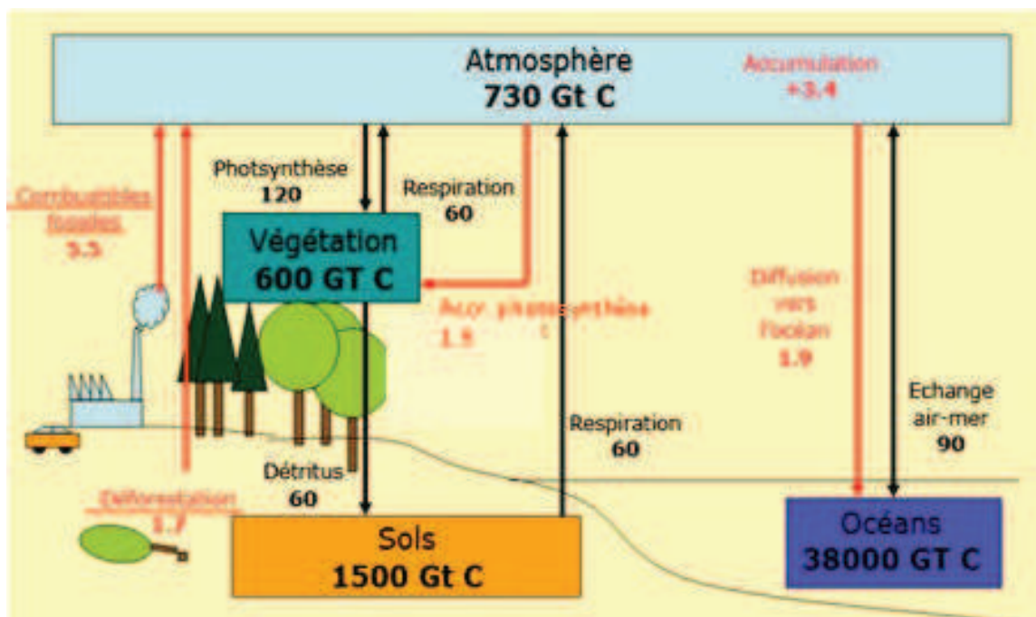
Doc. 4 : Les flux et les stocks de carbone dans le système Terre. En rouge et souligné, les flux supplémentaires liés aux activités humaines. Unités : Gt C (milliards de tonnes de carbone) par an.
